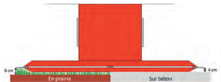
Figure 2. Réglages des couteaux d'une faucheuse à tambours, en prairie et sur béton
